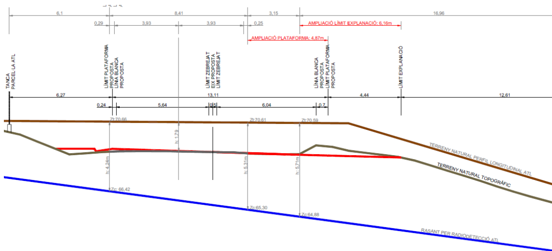
Figura 3. Superposició del terreny natural, la secció futura i la secció del terreny del plànol d'ATL.
