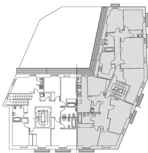
Planta primera
