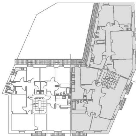
Planta tercera
